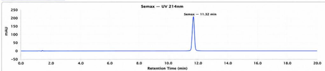
Semax 10mg - PS-SEMXX10005261 : UV Chromatogram
